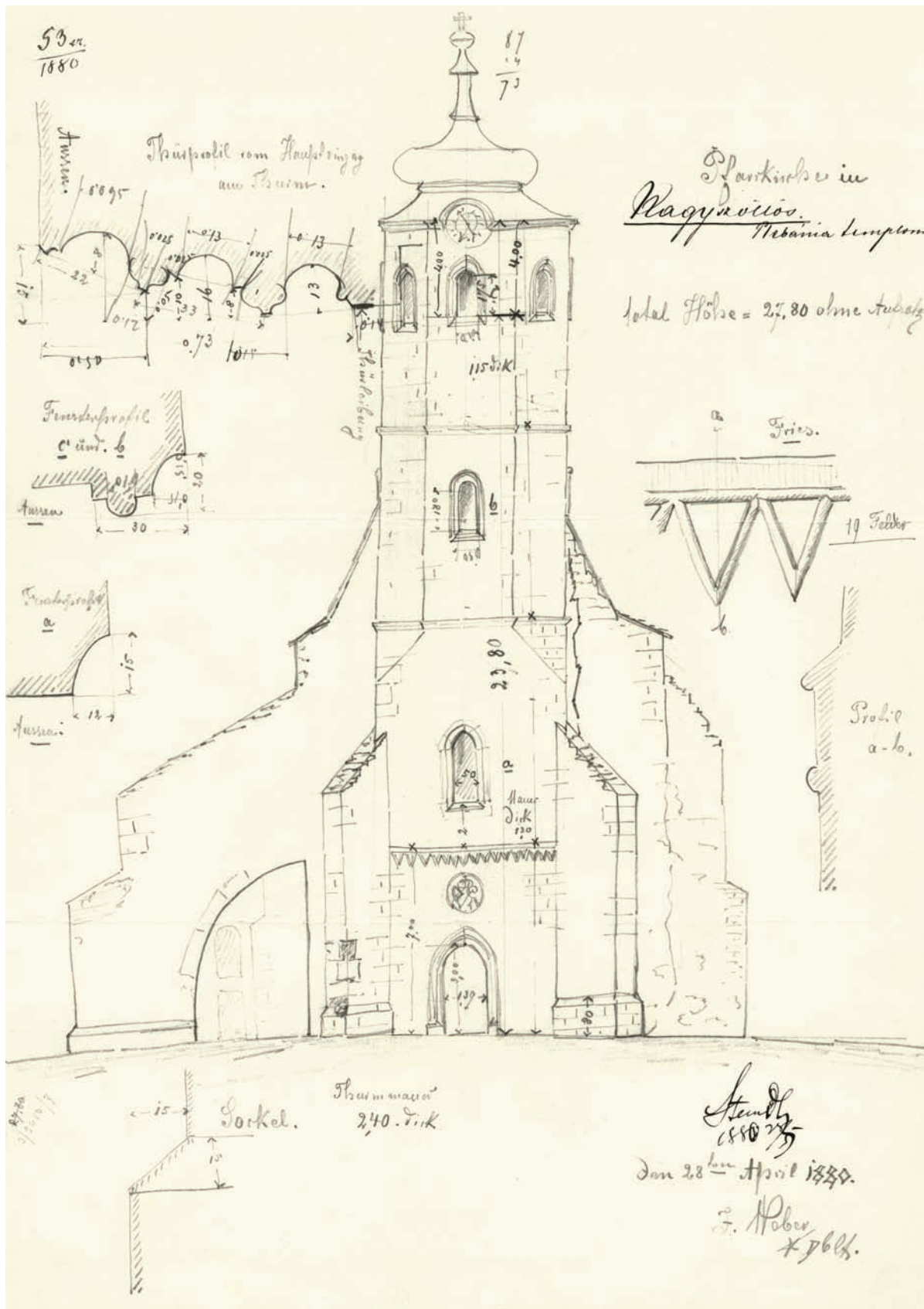
8. Західний фасад церкви з малюнками деталей (Г. Вебер, 1880 р.)
