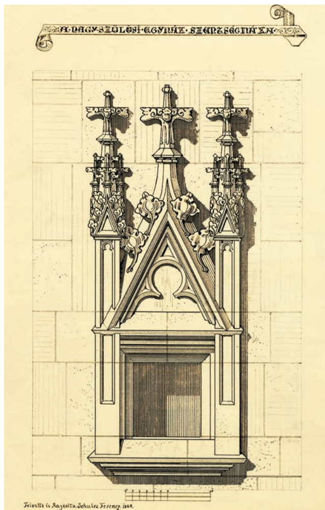
20. Обмір пастофорію (Ференц Шульц)
