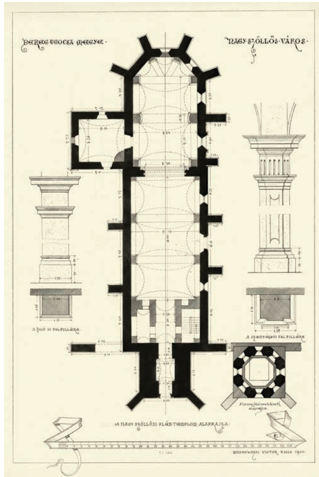
3. План церкви з деталями (Віктор Мишковський, 1900 р.)
