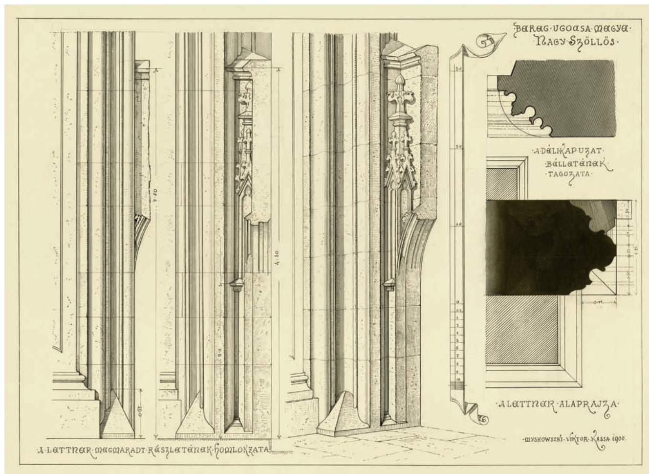
16. Обміри про залишені частини лекторіуму (Віктор Мишковський, 1900 р.)
