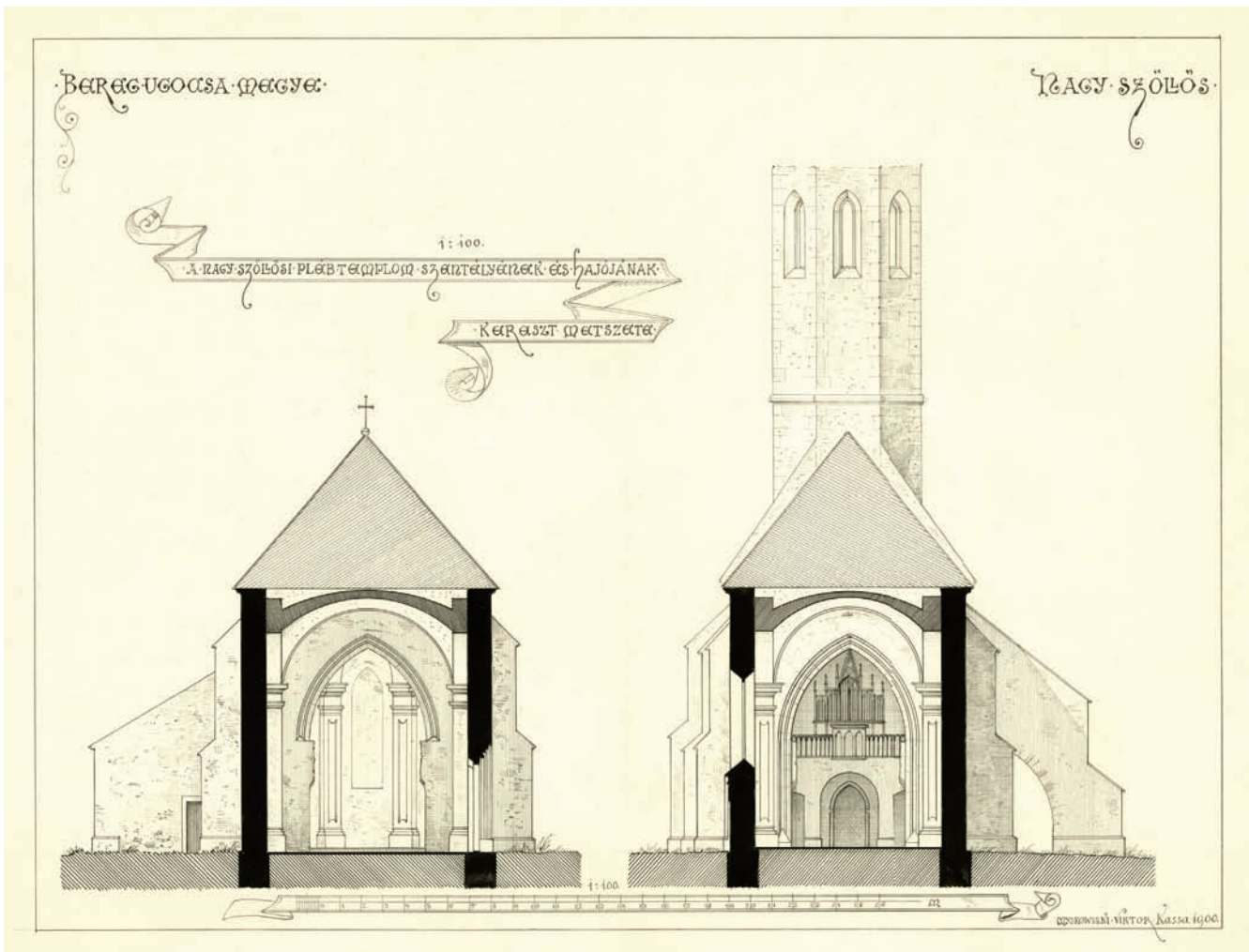
6. Поперечний розріз нефу та апсиди (Віктор Мишковський, 1900 р.)
