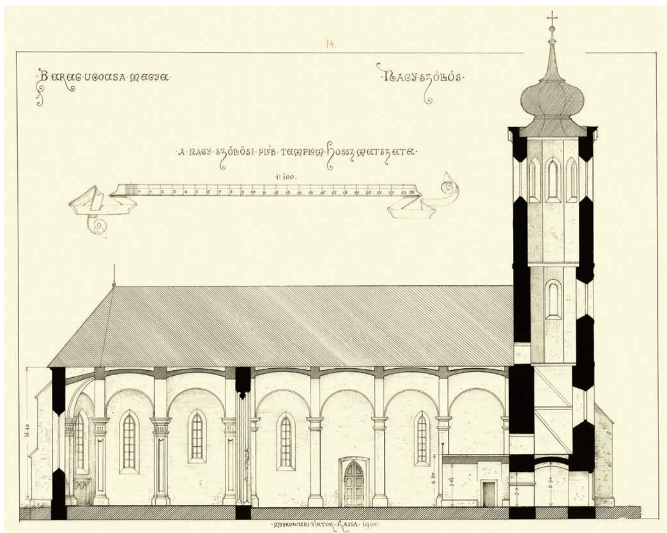
5. Поздовжній розріз церкви (Віктор Мишковський, 1900 р.)
